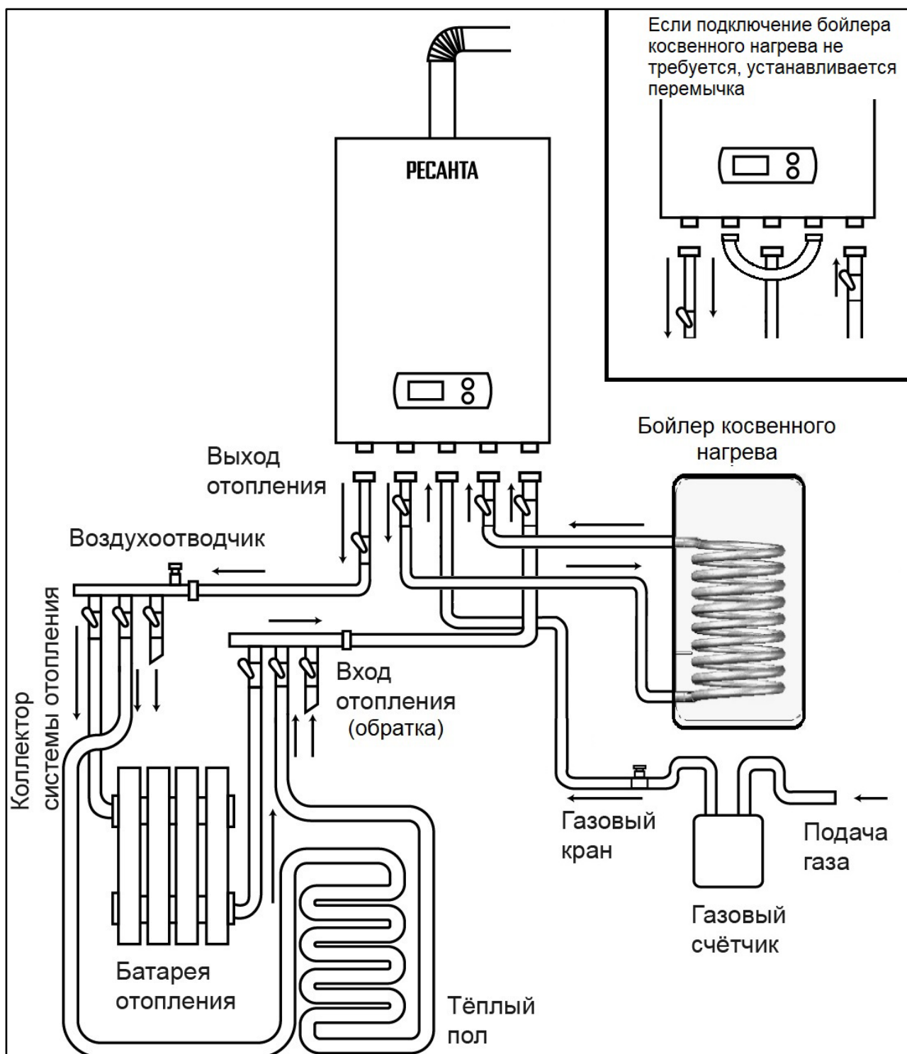
Рис. 7. Схема подключения газового одноконтурного котла
