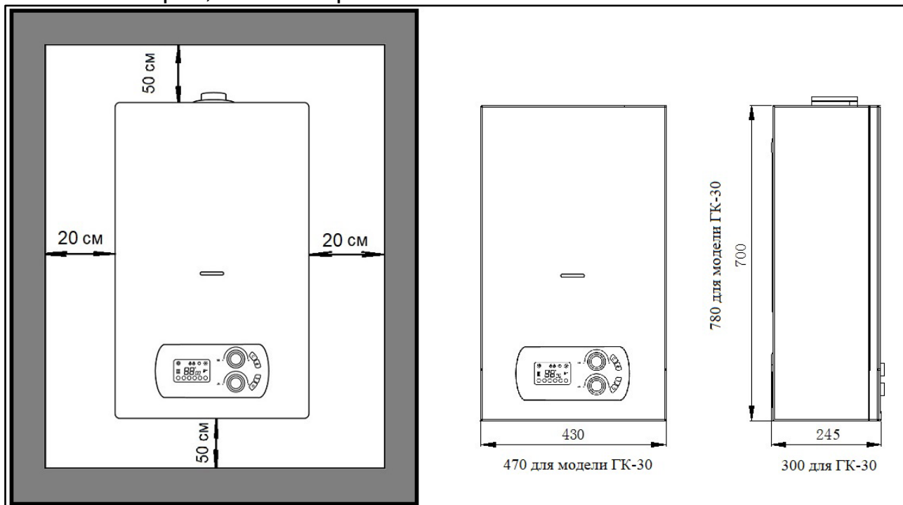
Рис. 3. Минимально допустимые расстояния и габариты котла
