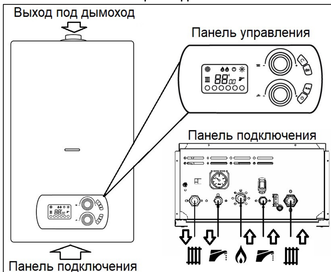
Рис. 1. Общий вид газового котла
