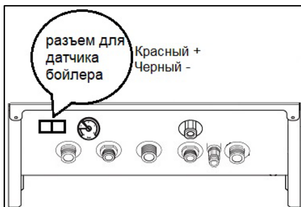
Рис.9 Разъем для подключения датчика бойлера.
