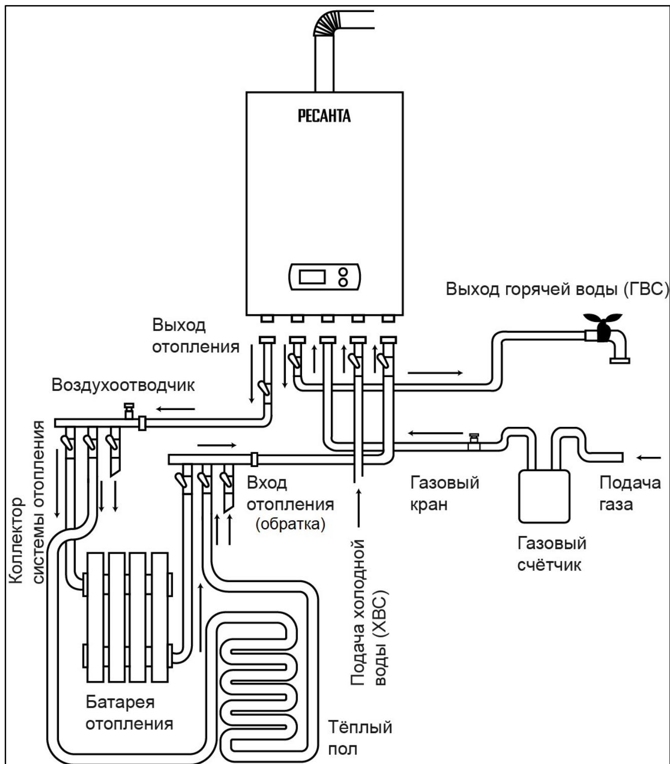
Рис. 6. Схема подключения газового двухконтурного котла
