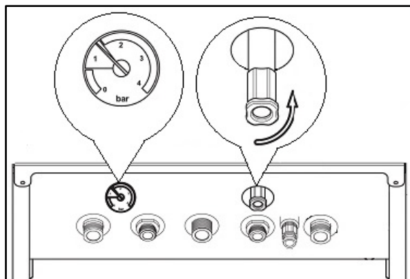
Рис.8 Кран подпитки и манометр
