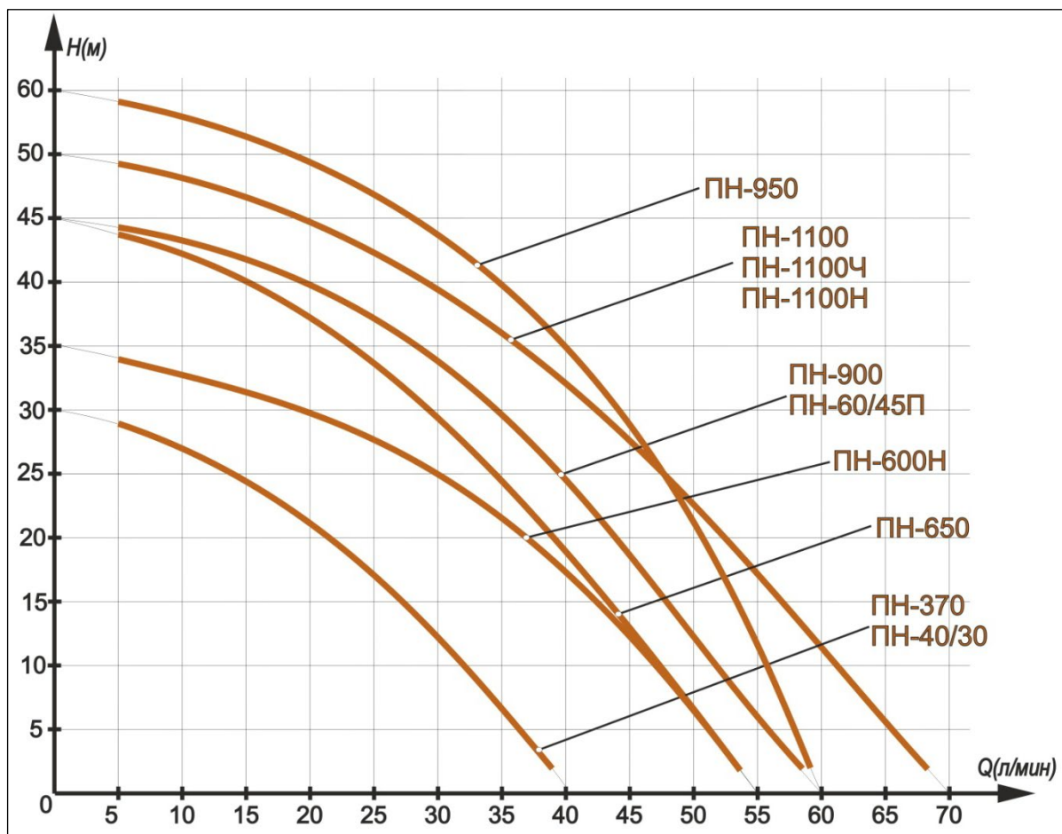
График 1 Напорно-расходная характеристика
