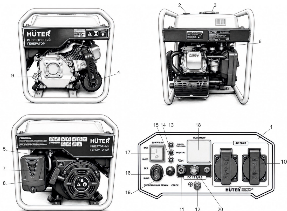
Рис. 2. Общий вид моделей DN 2700i, DN3700i, DN A3,7i GR, DN4400i, DN A4,4i GR, DN5500i, - DN 6500i-P, DN A6,5i-P GR.
