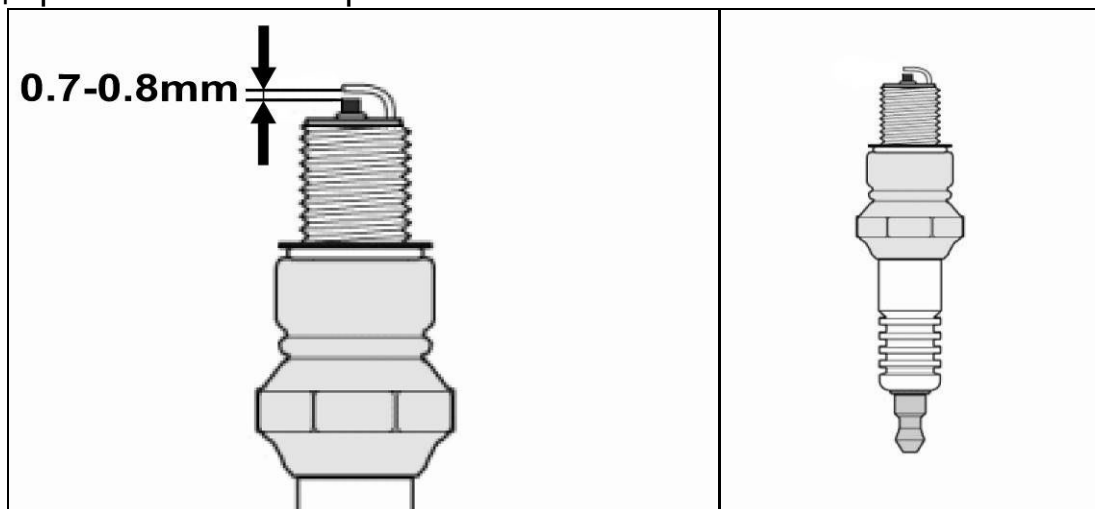
Рис. 15. Свеча зажигания
