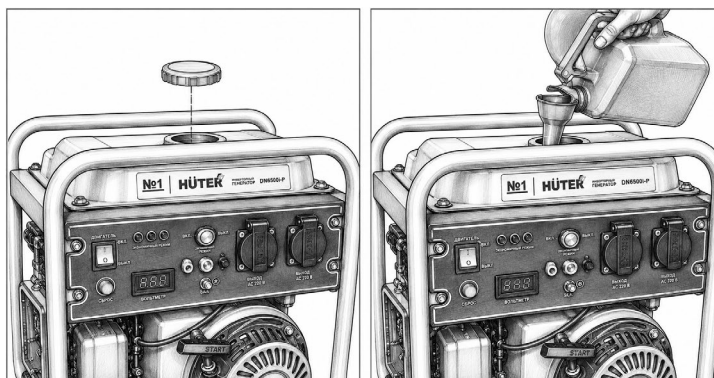
Рис. 7. Заправка бензином
