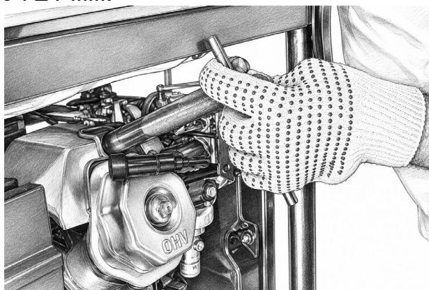
Рис. 14. Высоковольтный провод и свеча зажигания
