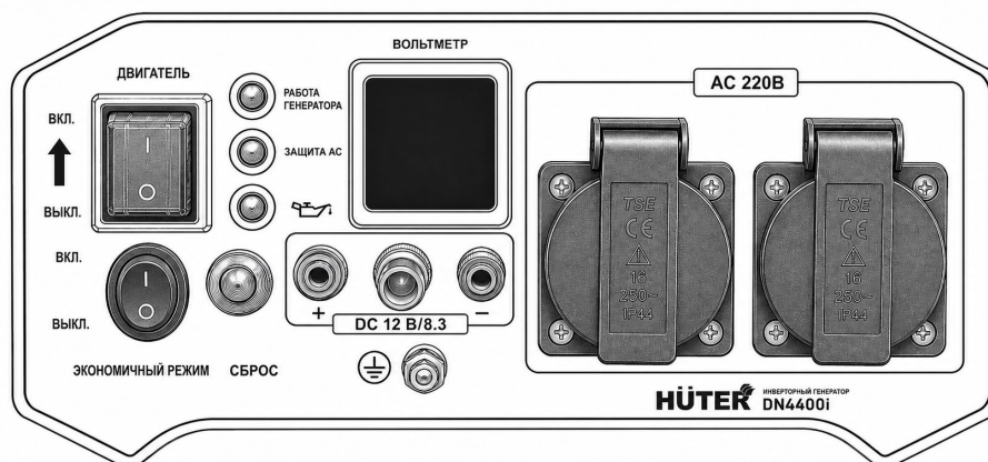
Рис. 11. Выключатель двигателя
