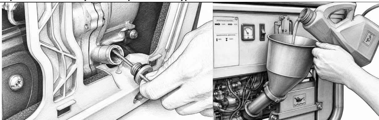
Рис. 4. Заправка маслом
