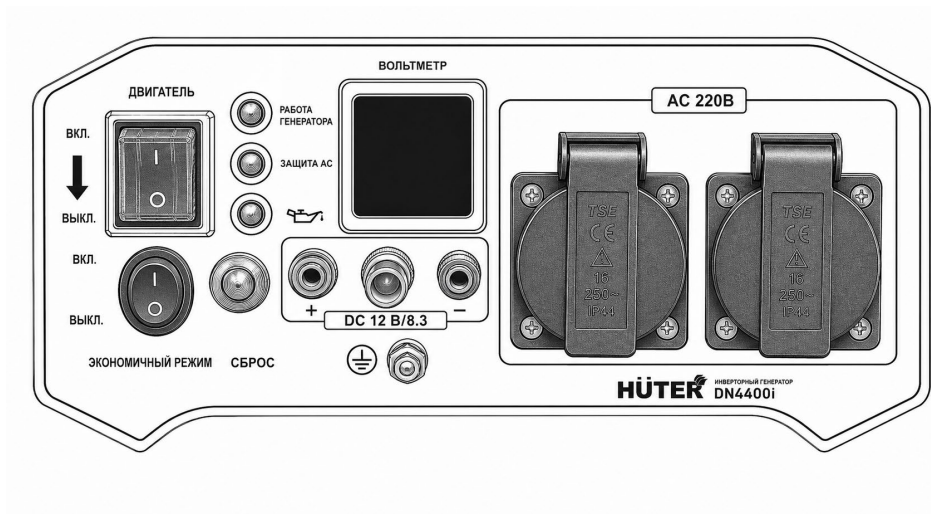
Рис. 10. Выключатель двигателя
