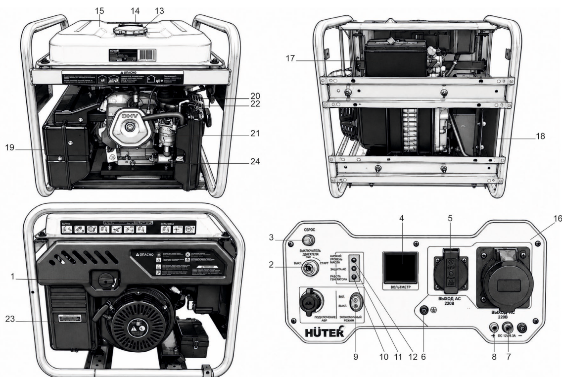
Рис. 3. Общий вид моделей DN7500i, DN A7,5i GR, DN12500i, DN12500iXA, DN A12,5iXA GR, DN13500iXA, DN A13,5iXA GR, DN19000iXA, DN A19,0iXA GR.
