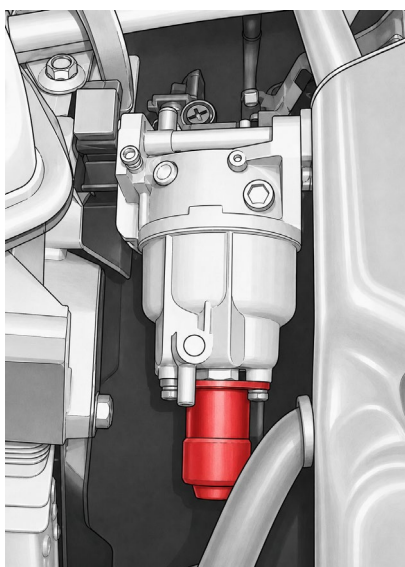
Рис. 18. Слив топлива из карбюратора
