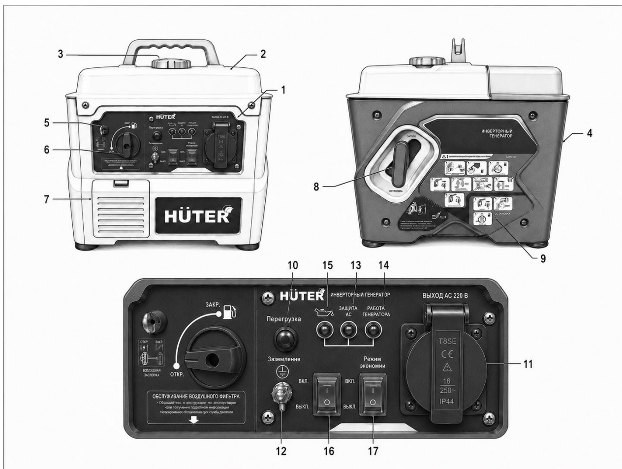
Рис. 1. Общий вид модели DN 1500i, DN A1,5i GR.
