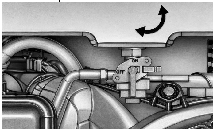
Рис. 8. Топливный кран
